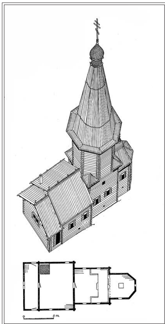
Космозеро. Успенская церковь (1720 г.). АксонOMETрия и план из книги Л. Петтерссона. Церковь ныне не существует.
